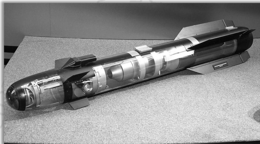
ตัวอย่างรูปภาพ จรวดอากาศสู่พื้น AGM-114 Hellfire (Wikipedia)
