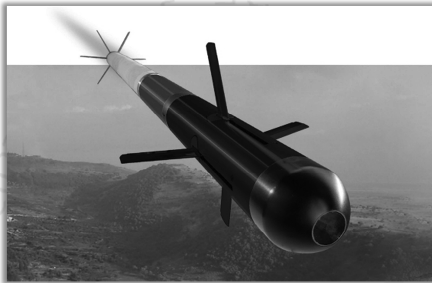
ตัวอย่างภาพร่าง จรวดนำวิถี GATR (Elbit Systems)
