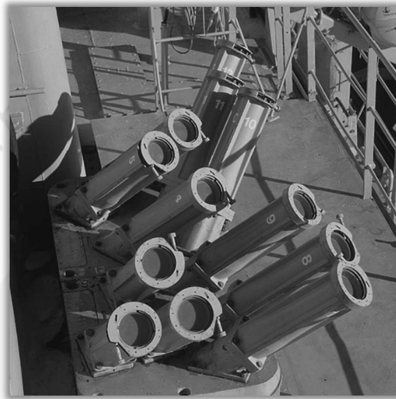
รูปภาพ ระบบเครื่องยิงเป้าลวง C-Guard Decoy (ที่มาของภาพ : Terma)
