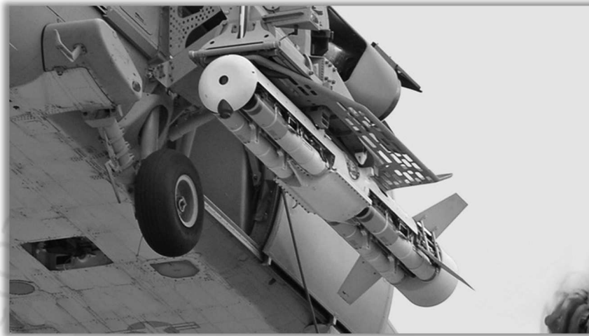
รูปภาพ ระบบทำลายทุ่นระเบิด Archerfish (ที่มาของภาพ : BAE Systems)
